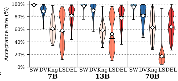
(d) Acceptance rate per sample.
